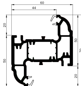
70mm Z Transom
