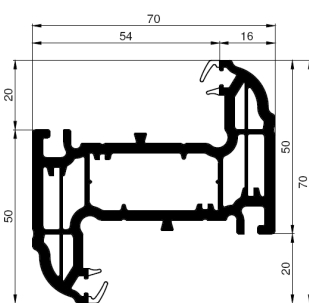
70mm Z Transom
