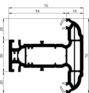
70mm T Transom
