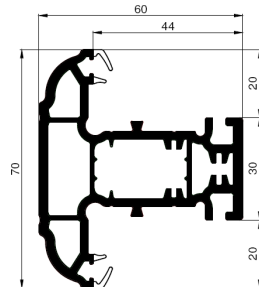
70mm T Transom
